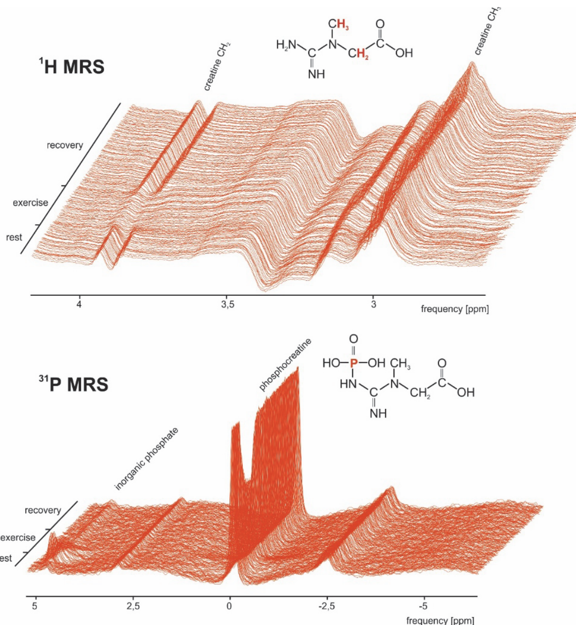
Obr.1: Reprezentatívny časový priebeh spektier ^1\text{H} (hore) a ^{31}\text{P} (dole) získaných počas 3 minút v pokoji, 5 minút cvičenia plantárnej flexie a 10 minút regenerácie z lýtkového svalu jedného dobrovoľníka. V štruktúrnych vzorcoch (P)Cr sú zvýraznené protóny a fosfor, ktoré spôsobujú signál MRS.
